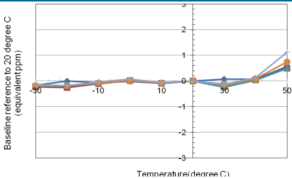
Baseline shift of NT-SO2-PL100
