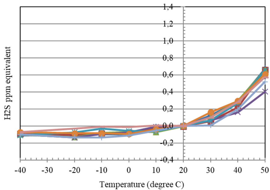
Baseline shift of NT-H2S-PL100
